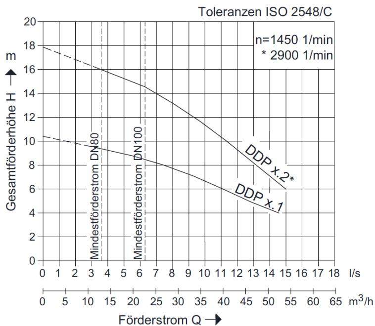
Bild 7: Pumpdiagram
